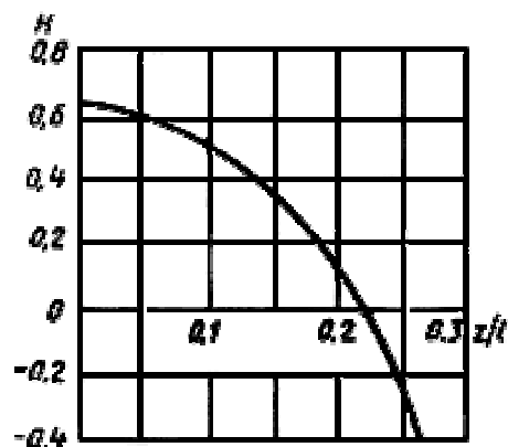
Рисунок В.1 - График для определения доли дисбаланса, подлежащего устранению в центральной плоскости коррекции
