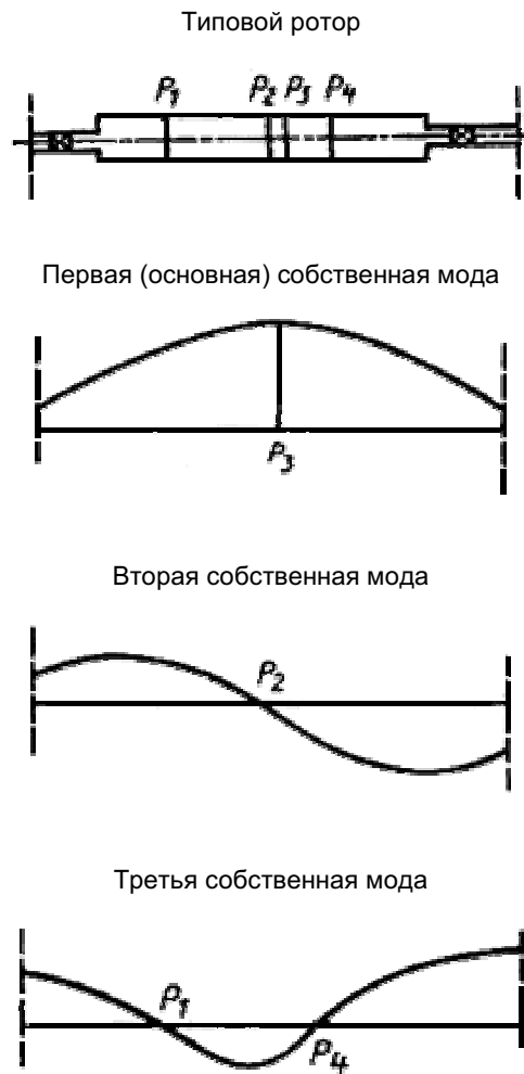
Рисунок 1 - Характерные собственные моды гибких роторов на податливых опорах
